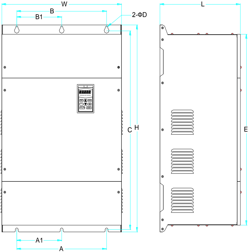
图 3: 壁挂式安装 (55KW-355KW)
