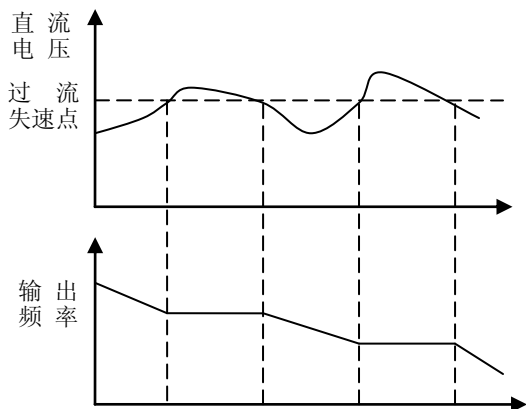
图 6-33 过压失速
